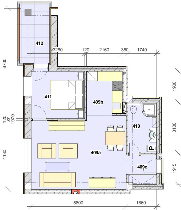
1 Apartmán č.402 1 : 100
