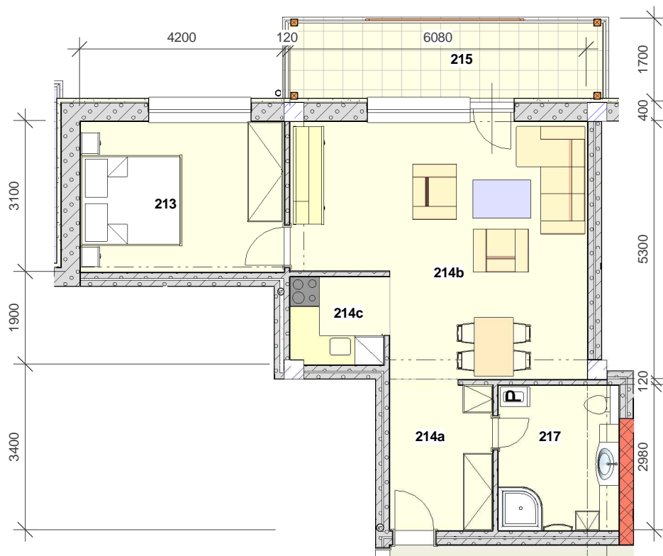
1 Apartmán č.203 1 : 100
