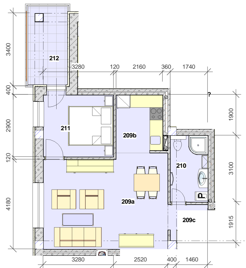
1 Apartmán č.202 1 : 100
