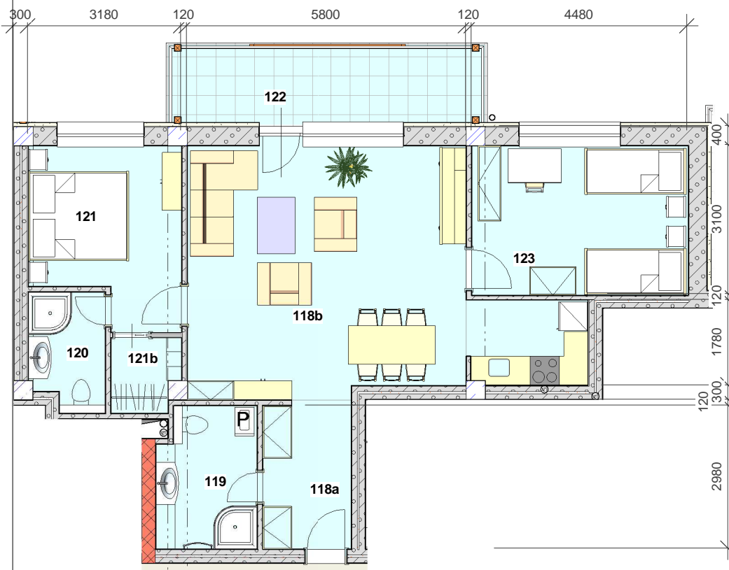
1 Apartmán č. 104 1 : 100
