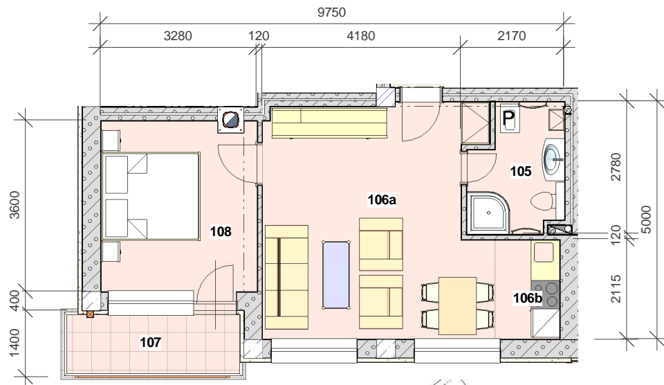
1 Apartmán č.101 1 : 100
